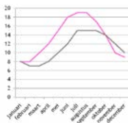
Ierland
